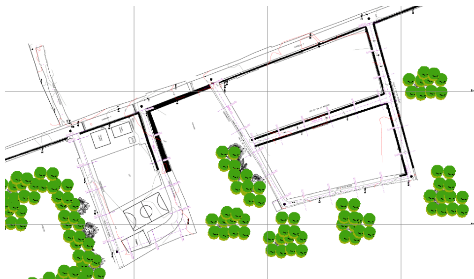
Imagen 4. Planta arquitectónica propuesta.
